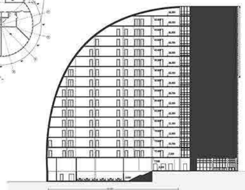
Разрез 1-1 M1:100
