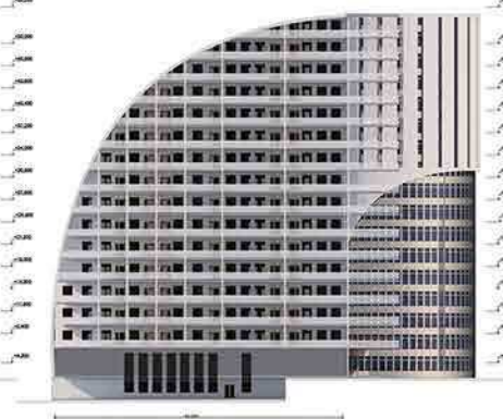
Фасад 6-1 M1:100
