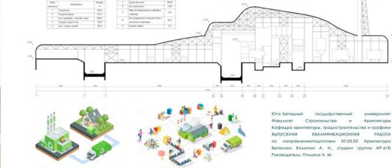
Разрез А-А М 1:200
