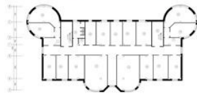
План на отм. 6,600 М 1:100
