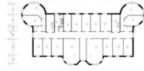
План на отм. 3,300 М 1:100
